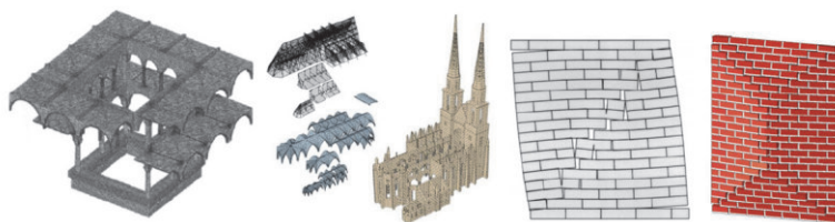
Slika 2. Primjeri modela i dosadašnjih istraživanja pristupom elemenata i njihove interakcije, redom [11, 16–18]
