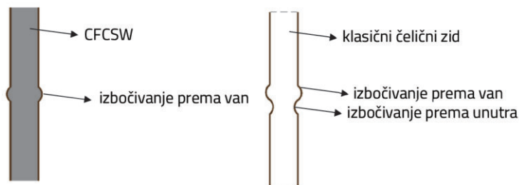
Slika 3. Način otkazivanja spregnutog i klasičnog čeličnog posmičnog zida, prilagođeno iz [8]
