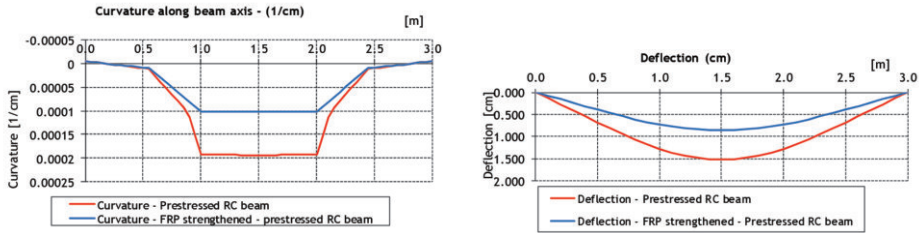
Slika 6. Usporedba M-1/r dijagrama i progibnih linija ojačane i neojačane grede
