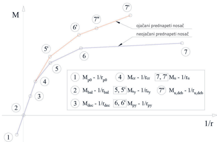
Slika 2. Usporedba M - 1/r dijagrama za pojačani i nepojačani presjek prednapete AB grede
